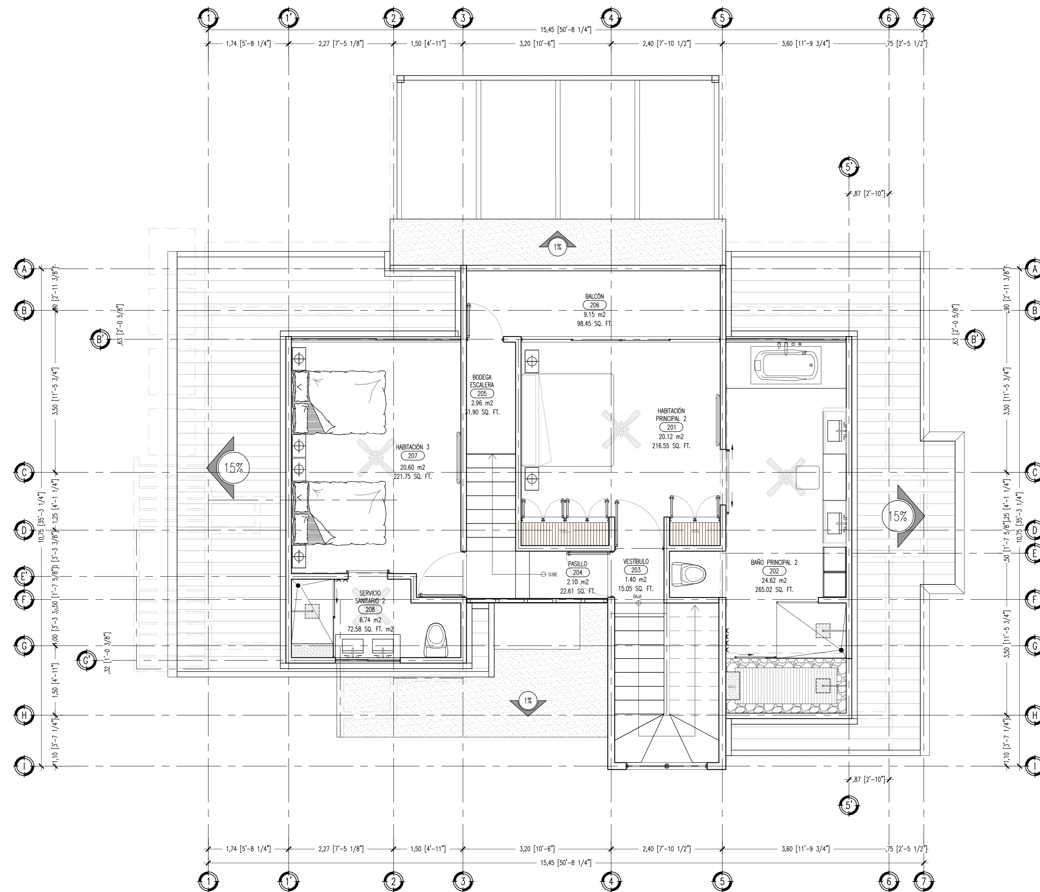
PLANTA ARQUITECTÓNICA DE DIMENSIONAMIENTO SEGUNDO NIVEL CASA 5 DORMITORIOS Escala 1:50
